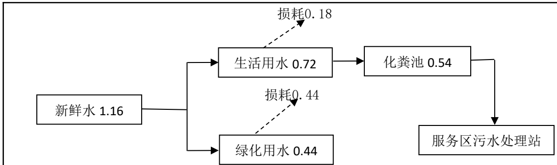
图 2 项目水平衡图 单位：m 3 /d
